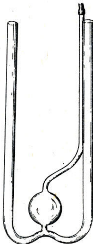
Рис. 16. Саморегулирующийся солевой обогреватель
