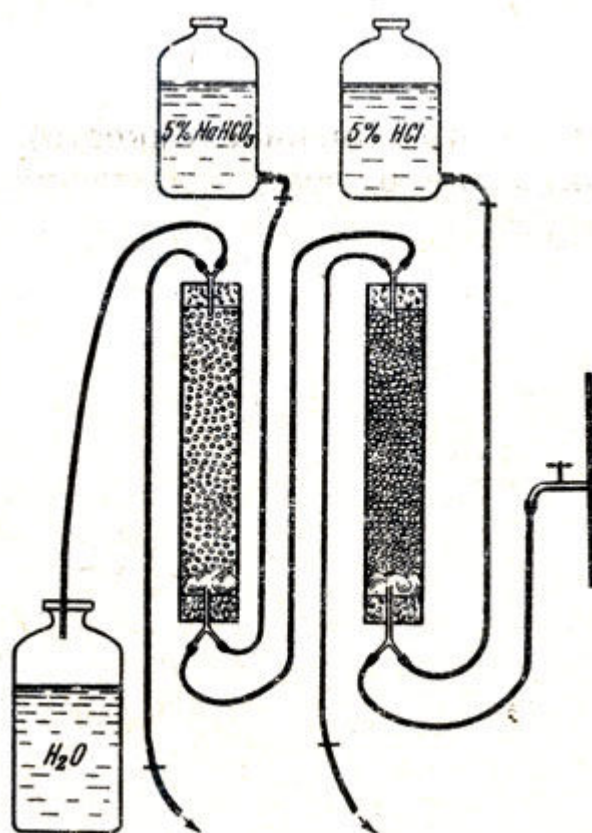
Рис. 66. Ионообменные колонки
