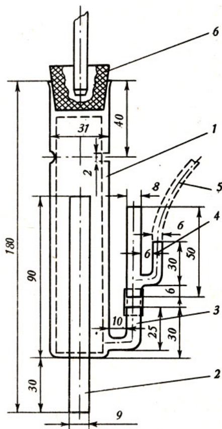
Рис. 26. Автоматический грязечерпатель
