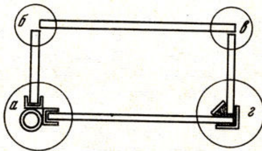
Рис. 6. Соединение стекол аквариума
