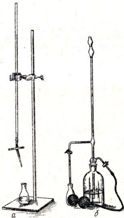
Рис. 65. Бюретка и микробюретка для тестирования
