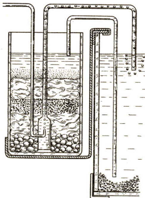
Рис. 22. Наружный фильтр
