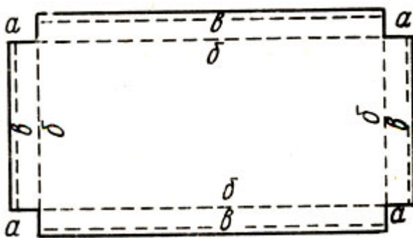
Рис. 4. Раскрой дна аквариума
