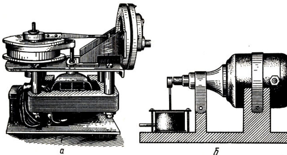
Рис. 19. Вибрационные компрессоры
