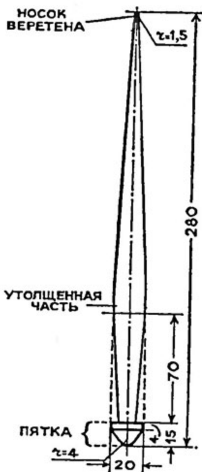
Эскиз веретена.
