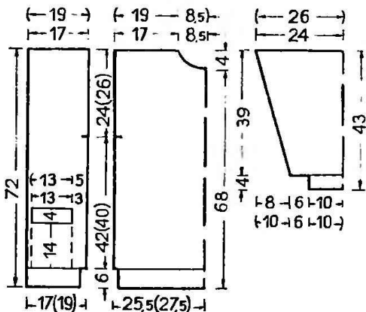
Чертеж выкройки жакета.
