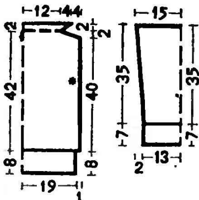
Чертеж выкройки детского пуловера: слева — \frac{1}{2} переда и спинки, справа — \frac{1}{2} рукава.
