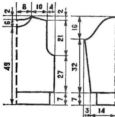
Чертеж выкройки костюма (размер 44—46).
