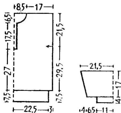
Чертеж выкройки женского пуловера (размер 46—48).
