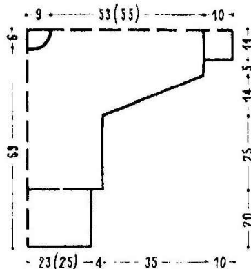
Чертеж выкройки макси-джемпера (размеры 42-44 и 46-48).
