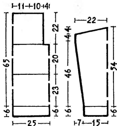
Чертеж выкройки мужского пуловера: \frac{1}{2} переда и спинки, \frac{1}{2} рукава.
