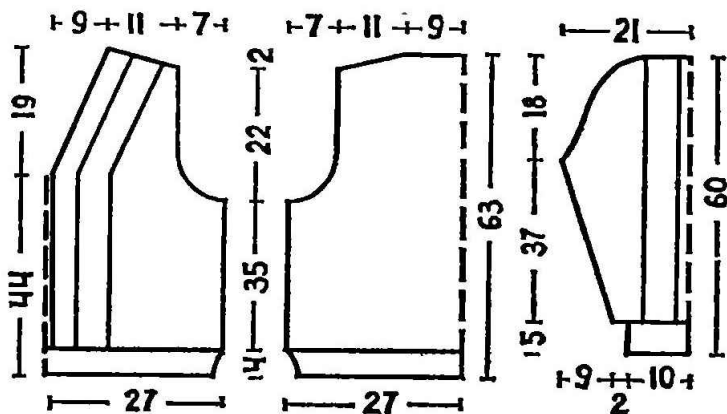
Чертеж выкройки пуловера (размер 50—52).
