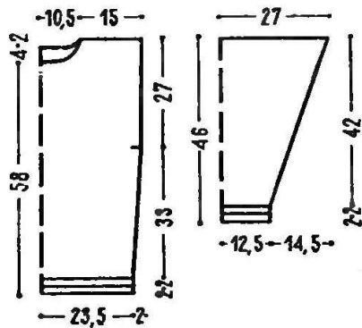
Чертеж выкройки пуловера с ажурными квадратами (размер 44—46).
