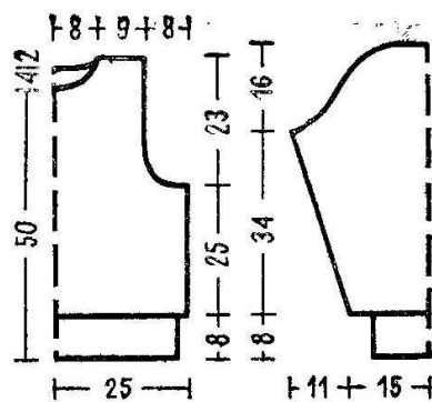
Чертеж выкройки пуловера с вышивной (размер 44—46).
