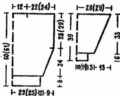
Чертеж выкройки свободного пуловера (размер 46—48).
