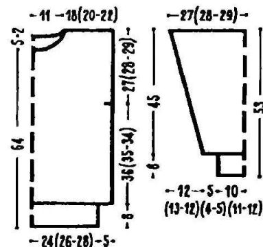
Чертеж выкройки мужского пуловера (размеры 48—50, 52—54 и 56—58).
